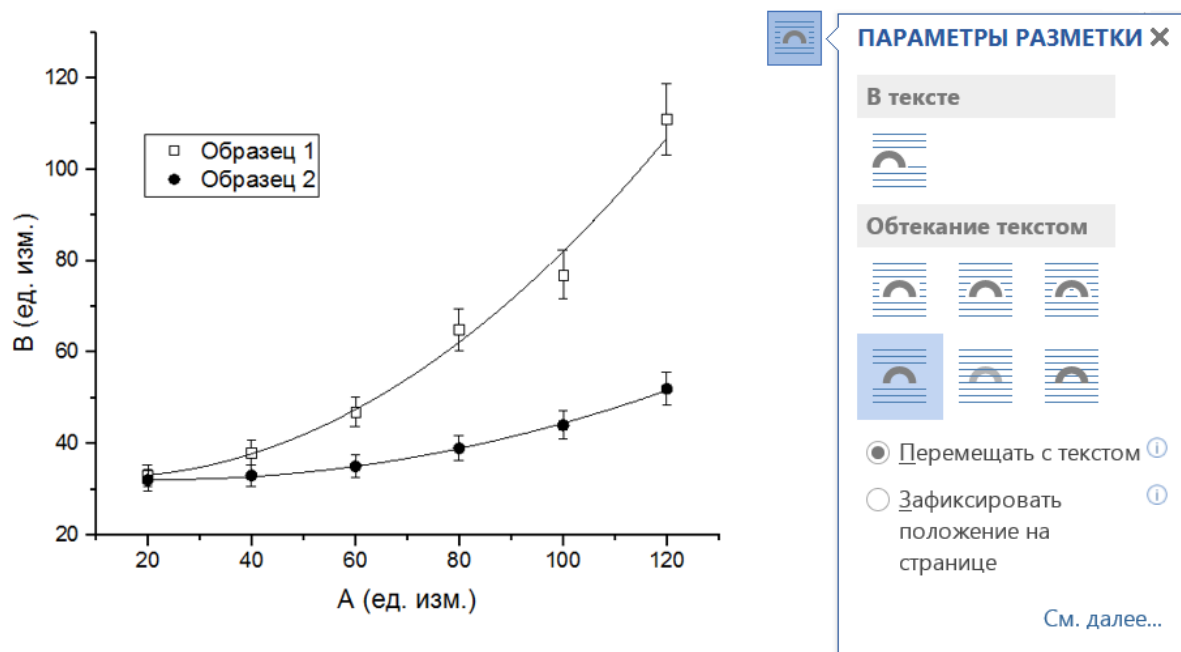
Рисунок 2.5 – Зависимость параметра B от параметра A для образцов 1 и 2. Сплошная линия – аппроксимация в рамках выбранной модели.
